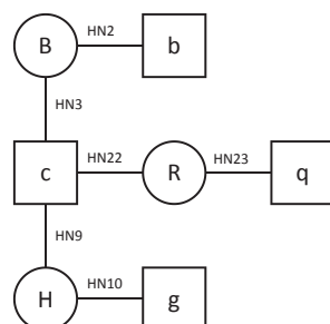
Kedja HS-Q3
